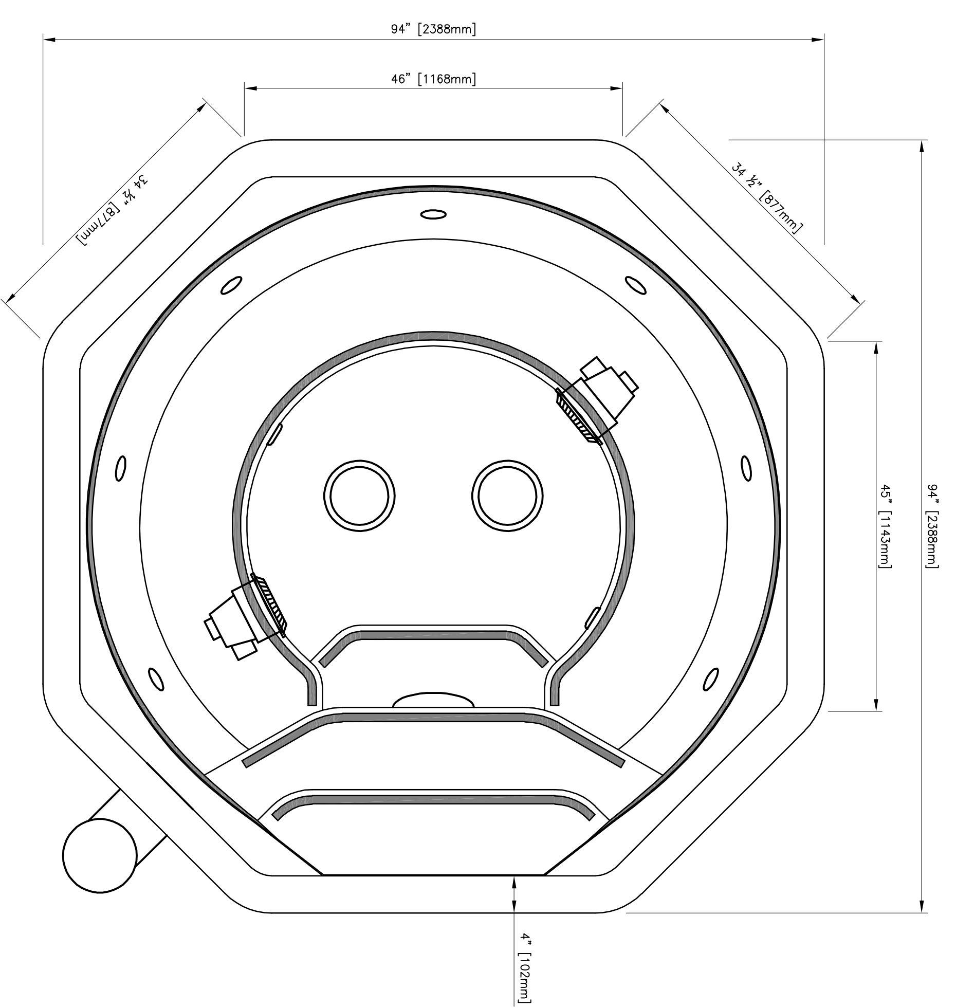
PLAN VIEW- SPA SCALE: 1"=1'-0"
