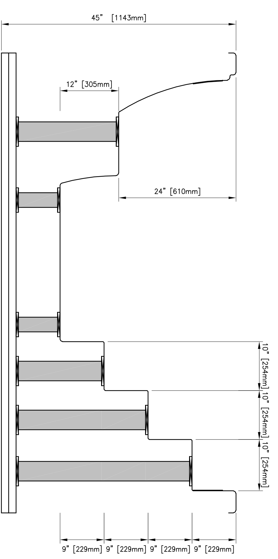
SECTION VIEW- SPA SCALE: 1"=1'-0"
